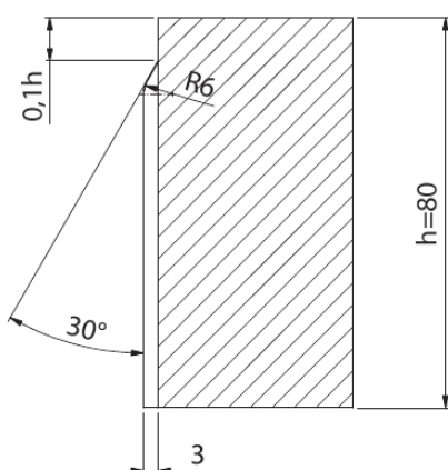
A-A (1:1)
