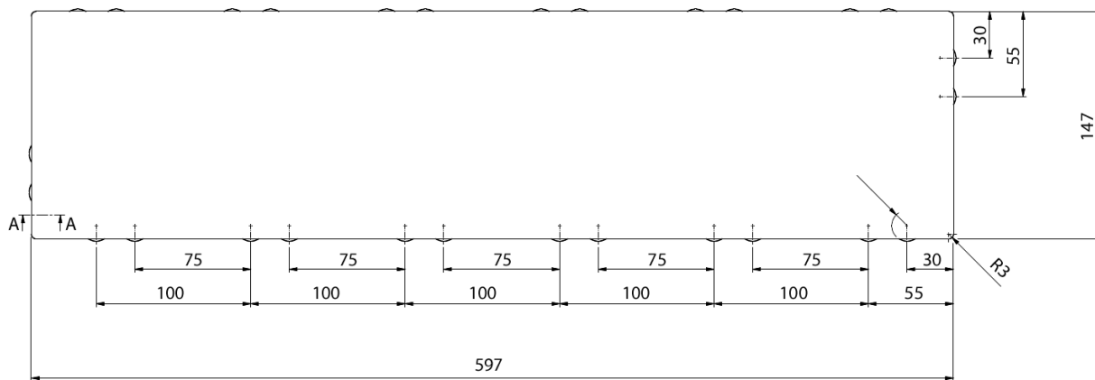
A-A (1:1)
