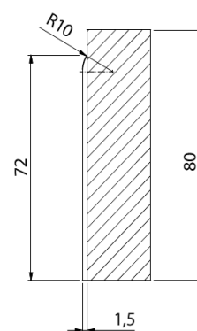
A-A (1:1)
